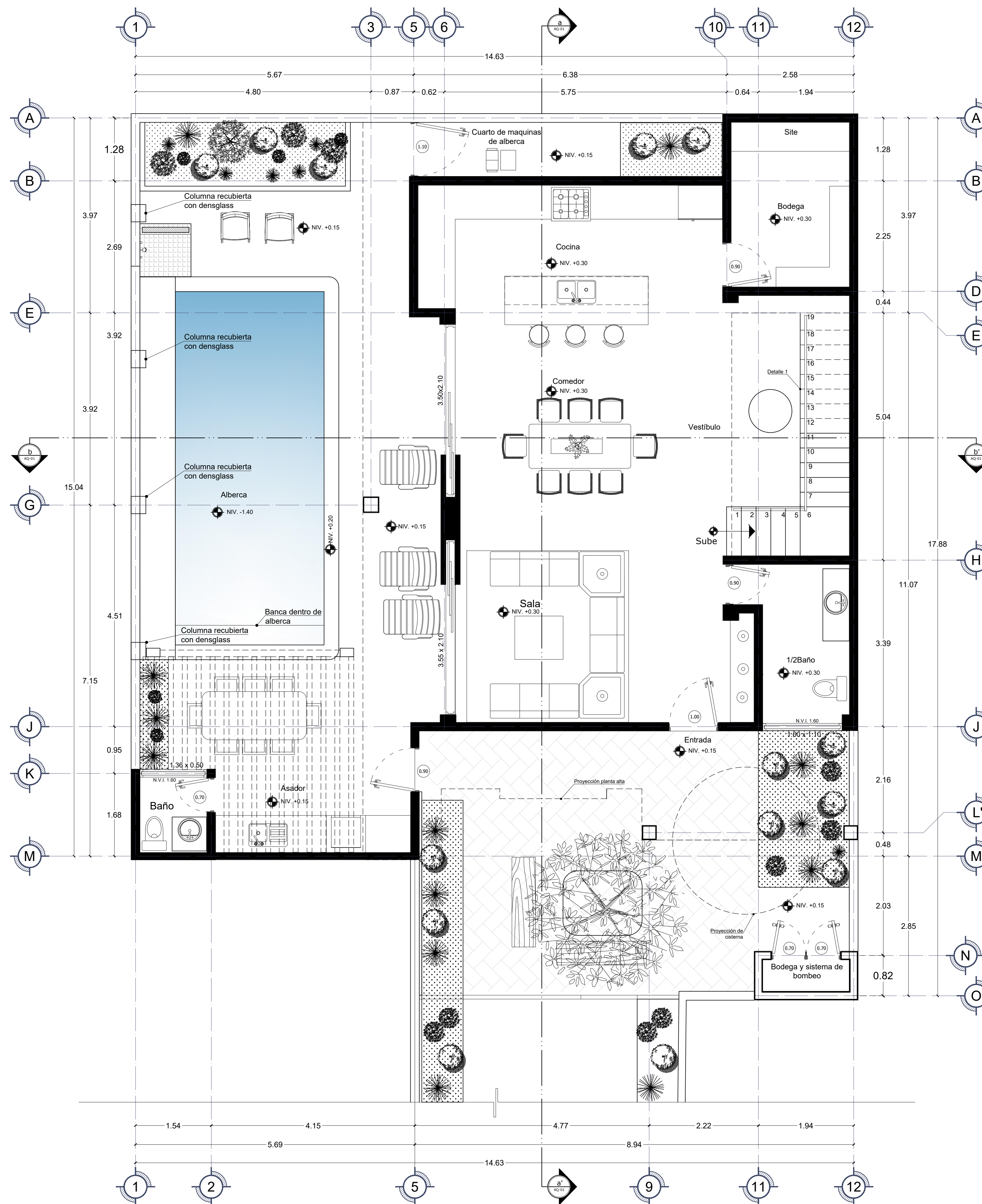
Planta arquitectónica baja Esc. 1:75 Área: 265.72 m 2
